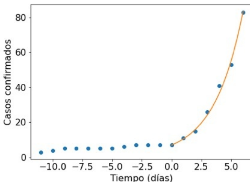
Figura 2. Evolución de la epidemia de coronavirus en México hasta el 16 de marzo, y ajuste a una curva exponencial de los datos a partir del 10 de marzo. El tiempo de duplicación del ajuste es de entre 1.66 y 1.69 días.
