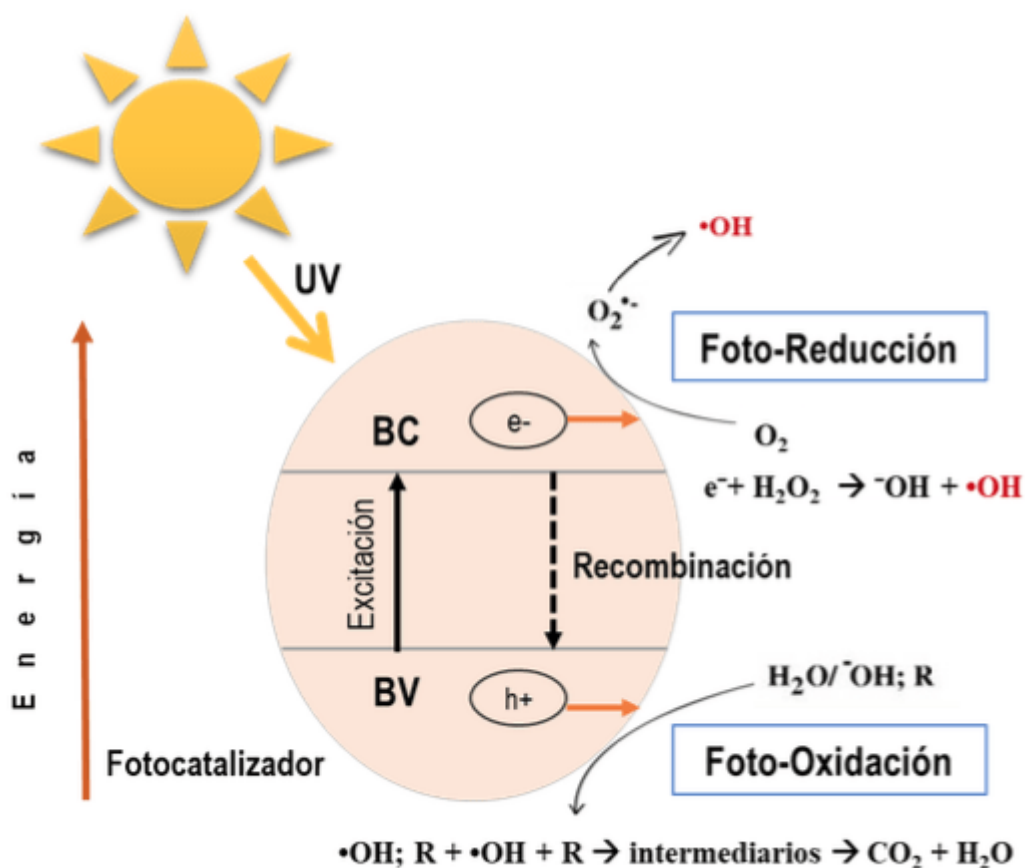
Figura 5. Representación del proceso fotocatalítico.
