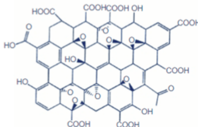
Óxido de grafeno
