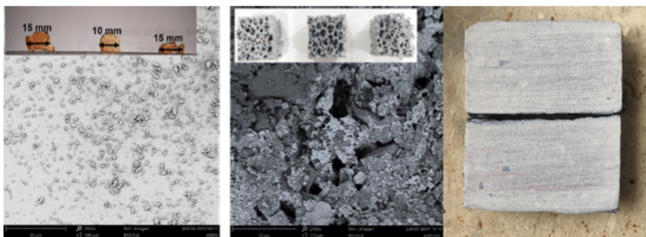
Figura 10. De izquierda a derecha, en la primera imagen se pueden apreciar monolitos de \text{SiO}_2\text{-WO}_3 , recubrimientos de \text{WO}_3 sobre espuma de SiC y \text{TiO}_2 "pintado" sobre barro cocido. [6]
