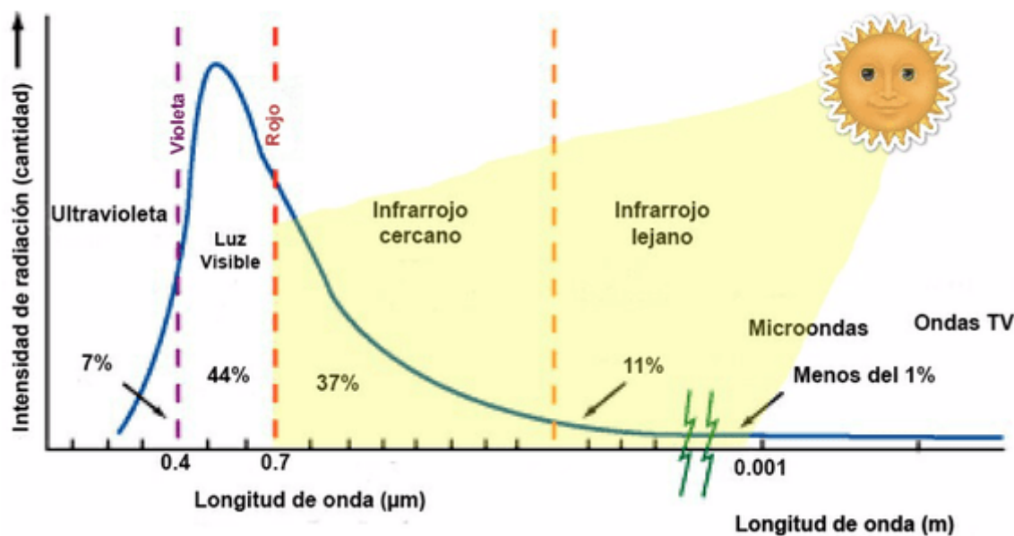
Figura 6. Espectro de radiación solar. Imagen modificada [8].
